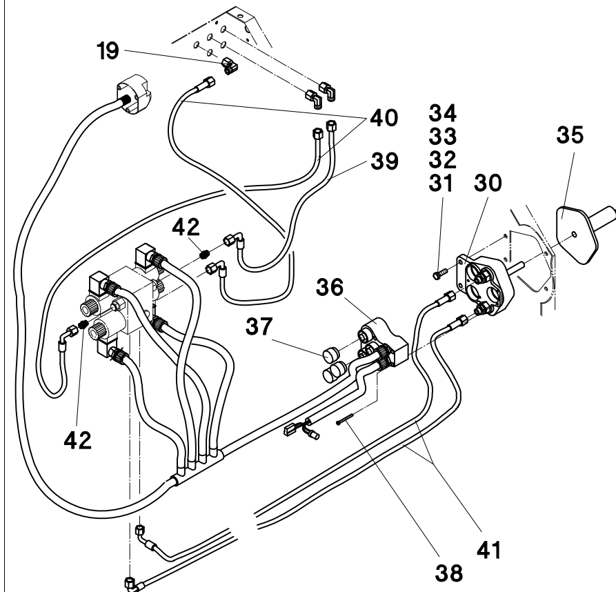
A (Pos.1-43)
